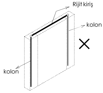
kayma çerçevesi modeli
